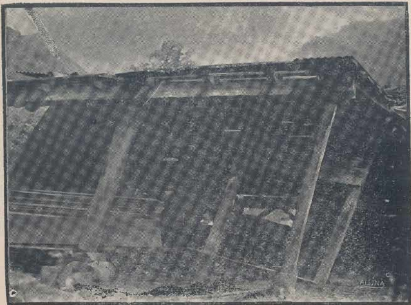
Esta casa de madera, que tenía techo mitad de tejas y mitad de zinc, fué parcialmente destruída. Conviene observar que estas construcciones que tenían techo de zinc ó de tablas de madera, fueron sólo dañadas ó movidas lateralmente de su posición primitiva.
